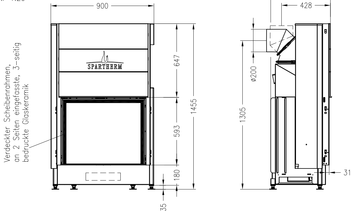
Vorderansicht M~1:20
